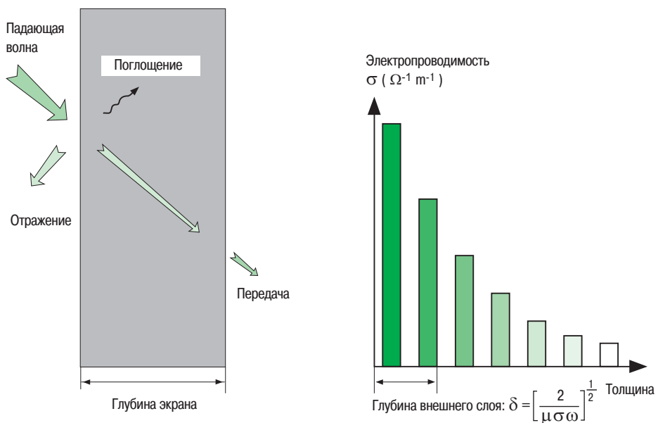
Рис. 19: Экранирующий эффект заключения в металлический кожух
