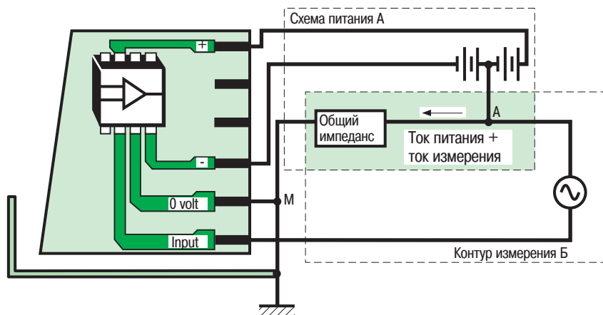
Рис. 13: Величины измеренные операционным усилителем будут неверны, потому что ток помехи в цепи А (электропитания) достаточно высок, чтобы создать напряжение помех в контуре В (измерение)
